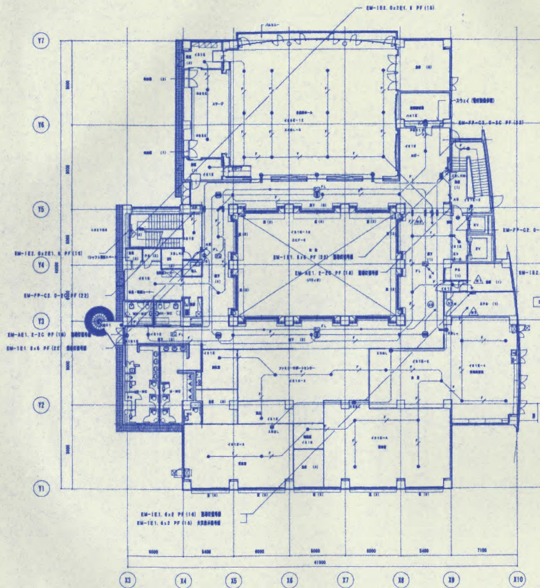
3階平面図 1/200
