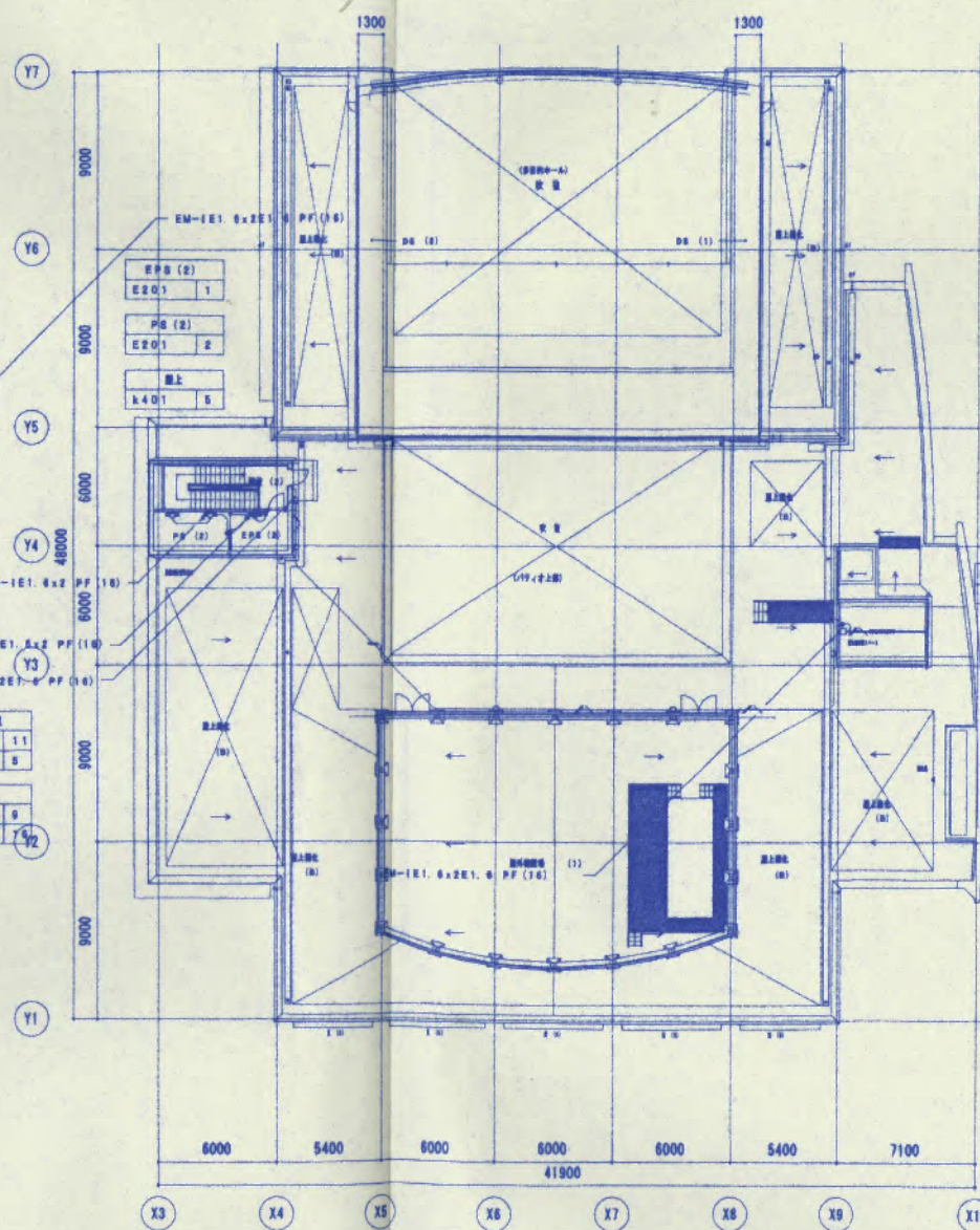
PH+3階平面図 1/200
